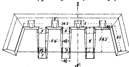
Профиль по линіи А-2.
