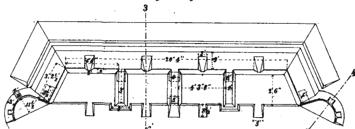
Профиль по линіи А-3.
