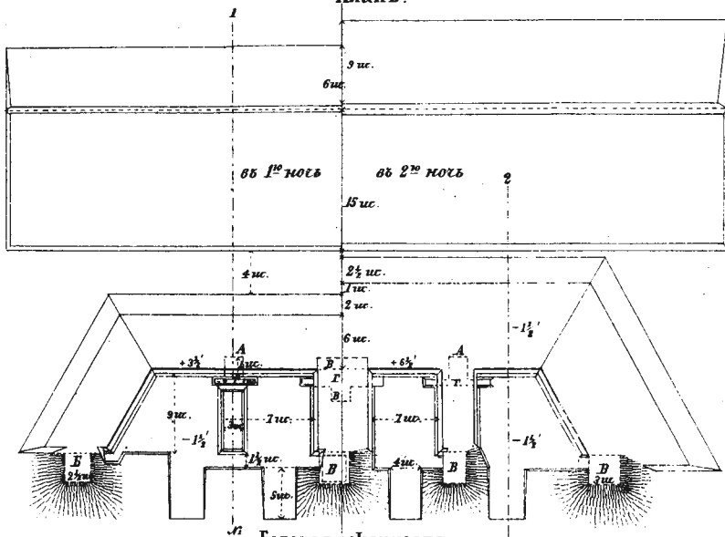
Фиг. 1. Нормальная осадная батарея. (Против крепости Карсъ летомъ 1877 г.) Планъ.
