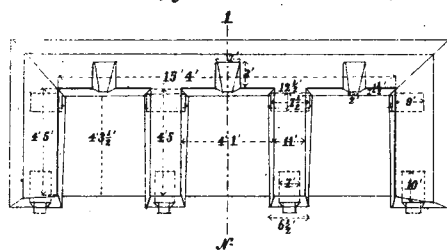
Профиль по линіи А-1.
